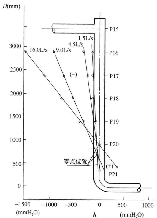
图 5 立管压力分布曲线 H —高度； P —测压点； h —压强
