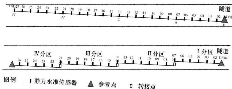
图2 静力水准线路分组安装示意图
