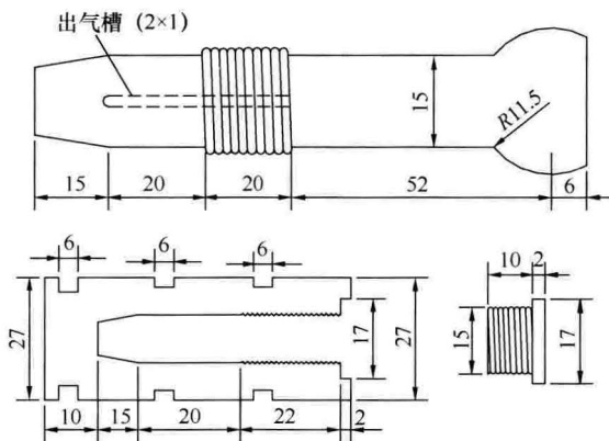
图 17 铸铁或不锈钢墙体暗标水准标志 (单位: mm)
