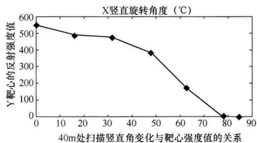
(b) 40m处扫描角度变化与靶心强度值的关系
