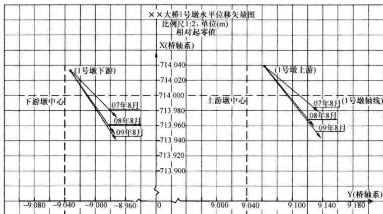
图 37 水平位移图
