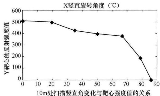
(a) 10m处扫描角度变化与靶心强度值的关系
