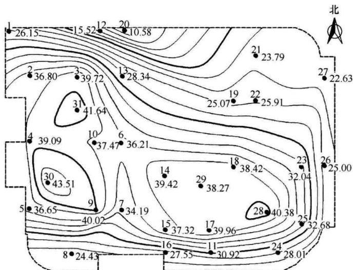
图 36 等沉降曲线
