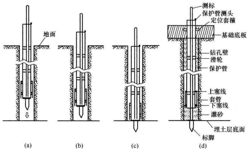
图 25 钻孔法埋设分层沉降标志
