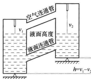
(a) 普通连通管式静力水准系统
