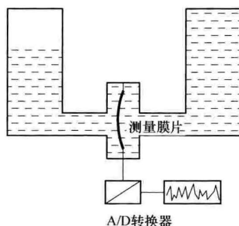
(b) 压力式静力水准系统
