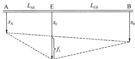
图 7.5.3 竖向的挠度
