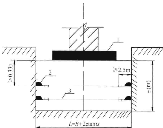
图 2 胞腔式固定方法
