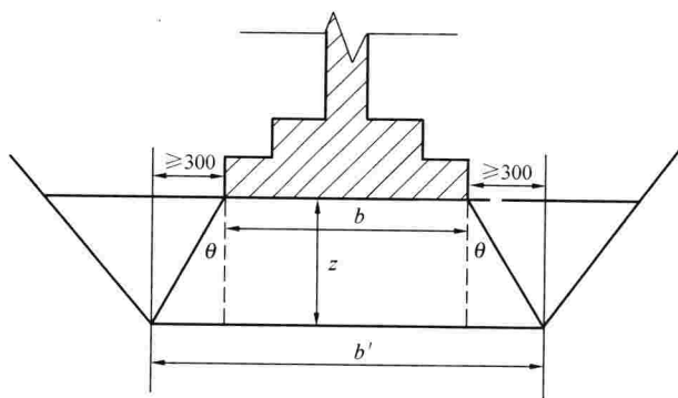
图 1 垫层宽度取值示意
