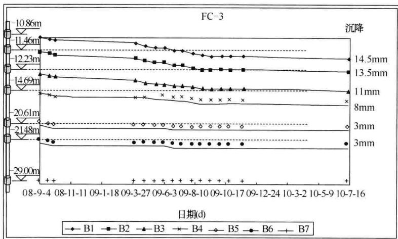
图 13 分层沉降变形曲线
