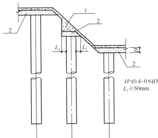
图 11 井坑斜面部位褥垫层做法示意图
