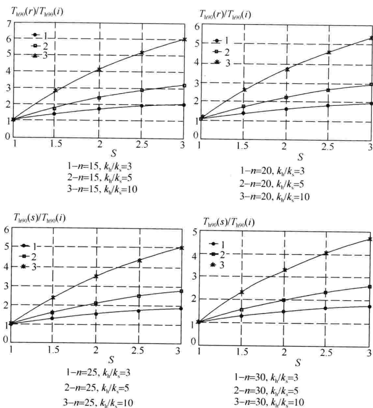
图4 涂抹对土层固结速率的影响
