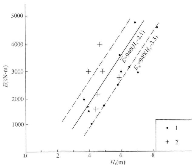
图7 夯击能与实测置换深度的关系
