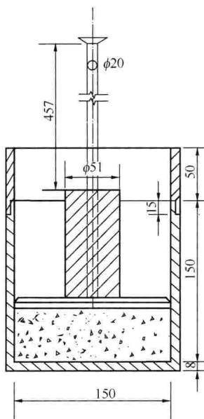
图 10 击实试验 主要部件示意
