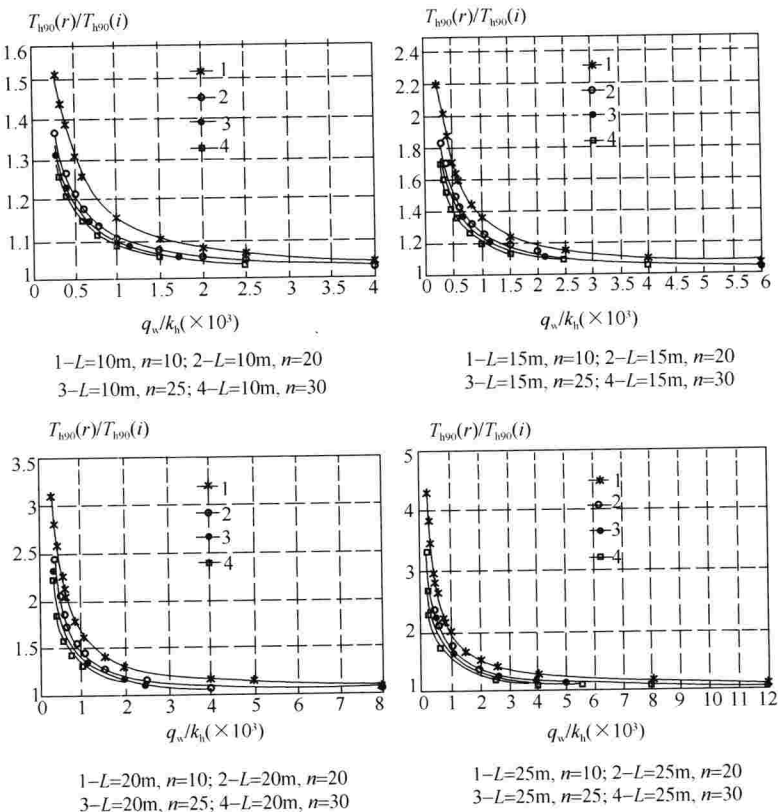
图5 井阻对土层固结速率的影响
