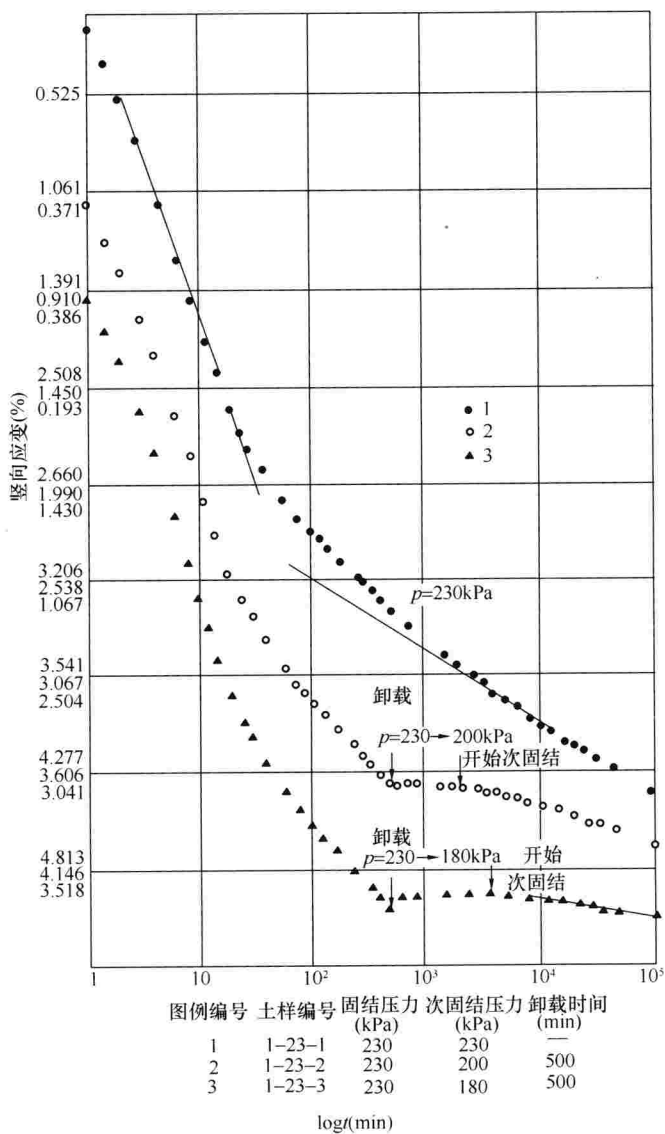
图 6 某工程淤泥质黏土的室内试验结果
