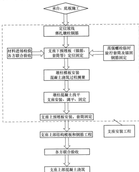
图2 支座安装的施工流程
