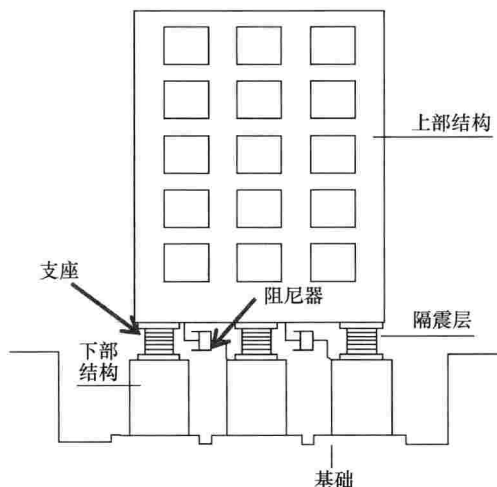
图 1 建筑隔震工程各部分示意图
