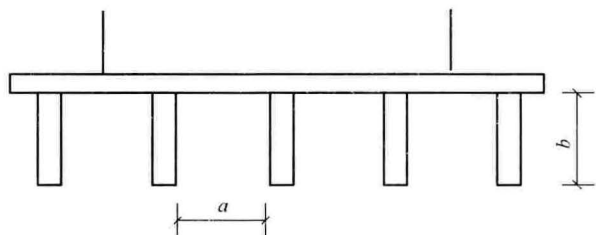
图 17 通透性吊顶的设置要求
