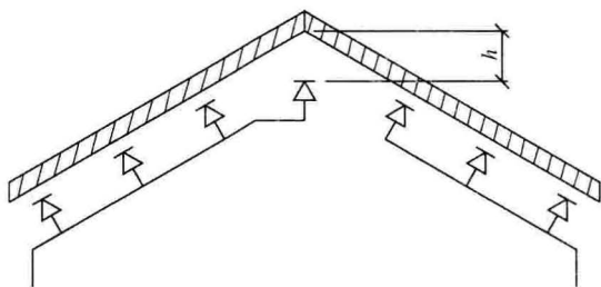
图 18 屋脊处设置喷头示意图
