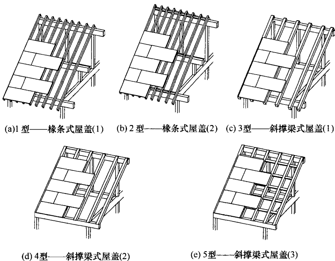
图 P.0.2 屋盖结构形式类型示意
