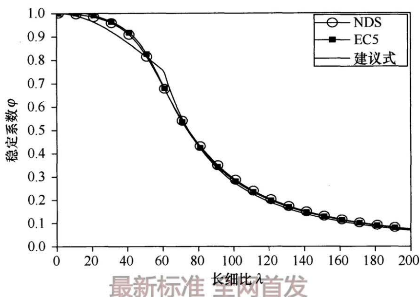
图 7 层板胶合木受压构件稳定系数比较 (TCT24)
