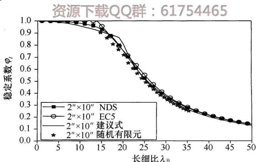
图 9 北美锯材受弯构件侧向稳定系数比较 (SPF No. 2 2"×10")
