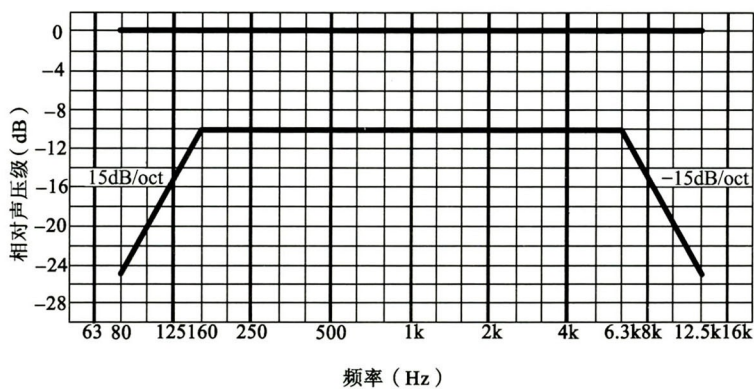
图 3.3.1-1 一级业务广播、一级背景广播室内传输频率特性容差域
