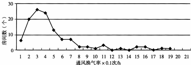
图 1 房间数按通风换气率大小分布(2016 年)
